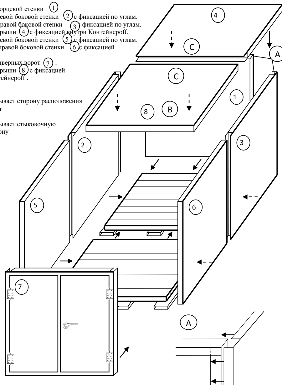
Рис. 1 Схема сборки Контейнерoff 4м
